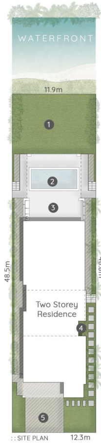
:: SITE PLAN THE BOULEVARDE
